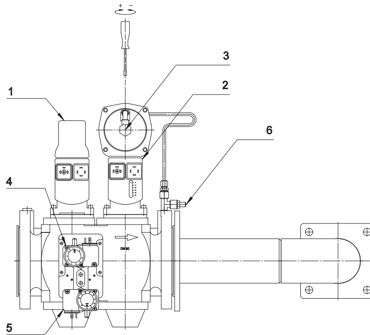
Fig. 15 ОСНОВНАЯ ГАЗОВАЯ ПАМПА: SIEMENS VGD40...
