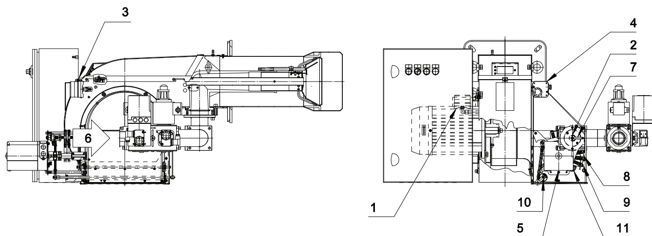
Fig. 8 РЕГУЛИРОВКА ГОРЕЛКИ
