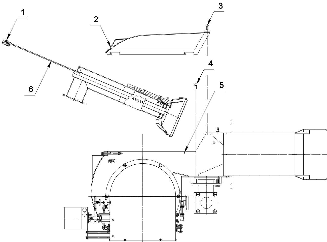
Fig. 31 ИЗВЛЕЧЕНИЕ СМЕСИТЕЛЬНОЙ КАМЕРЫ
