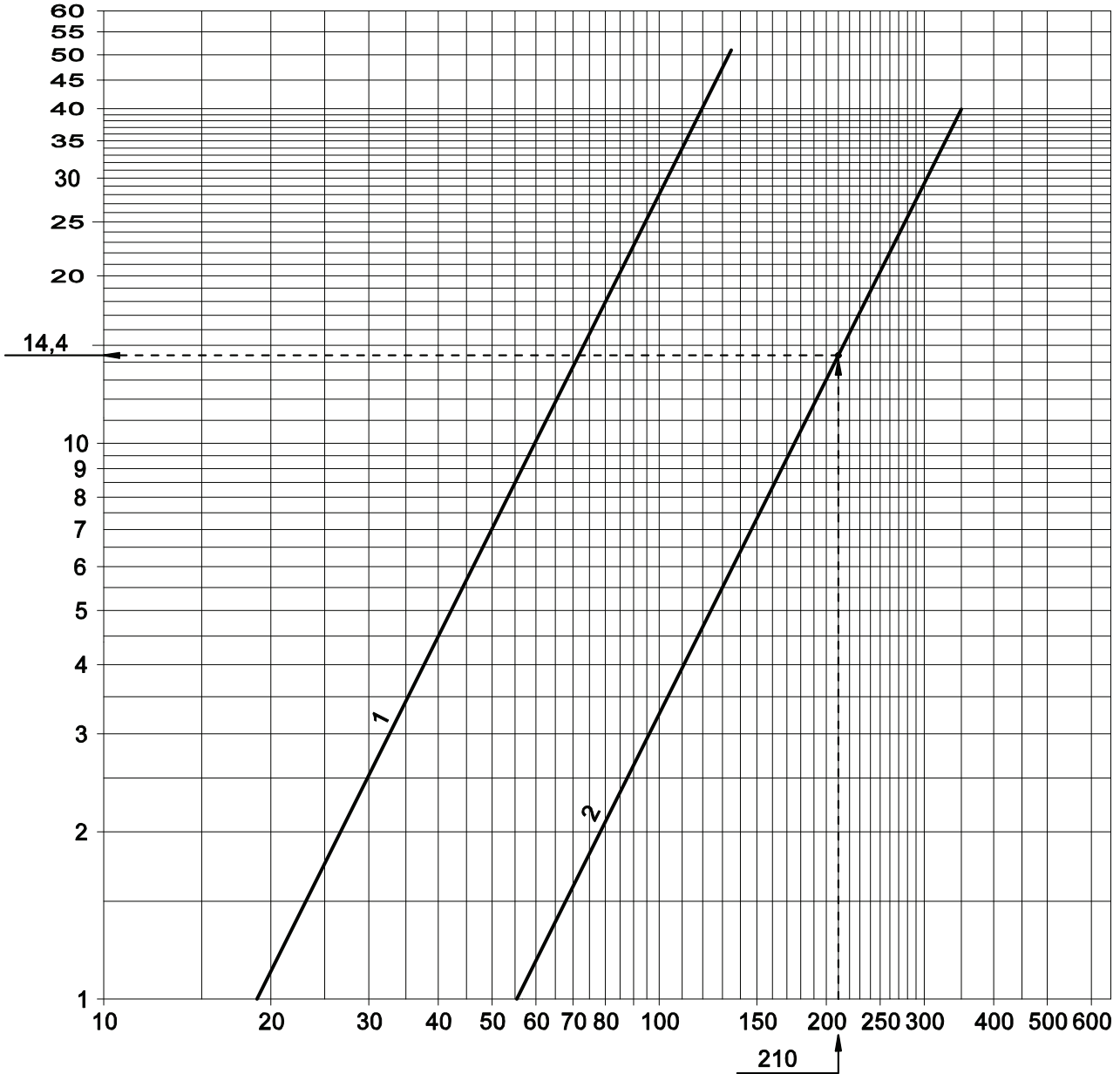
Fig. 29 Ось X= РАСХОД ГАЗ [мЗ/час] ; Ось Y= P: давление график [мбар]
